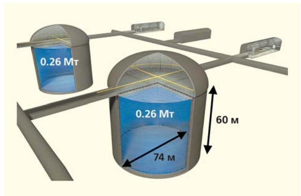
Рис.7. Установка HyperKamiokande, состоящая из двух черенковских детекторов — гигантских цистерн, заполненных чистой водой. Черенковское излучение регистрируется большими фотоумножителями, расположенными по всей внутренней поверхности цистерн. Масса воды в каждой цистерне составляет 0.26 Мт.
