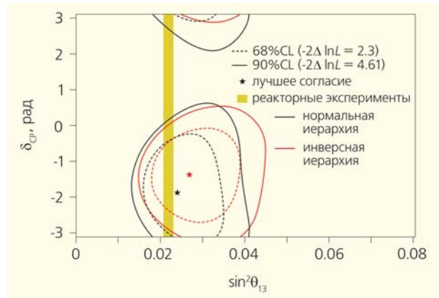
Рис.3. Области значений \sin^2\theta_{13} и \delta_{CP} , полученные в эксперименте T2K при измерениях вероятностей осцилляций мюонного нейтрино (в электронное нейтрино) и мюонного антинейтрино (в электронное антинейтрино). Пунктирная кривая показывает интервал параметров, соответствующий доверительному интервалу (CL) 68%, сплошная кривая соответствует 90% CL. Показаны результаты для нормальной и инверсной иерархии масс. Сплошная вертикальная полоса показывает \pm 1\sigma интервал значений \sin^2\theta_{13} , измеренных в реакторных экспериментах.
