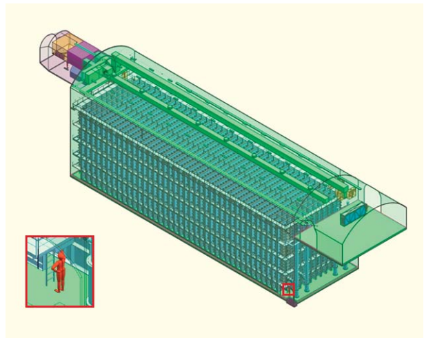
Рис.6. Схематическое изображение одного из модулей (время-проекционной камеры, заполненной жидким аргоном) эксперимента DUNE. Примерные размеры модуля: длина около 60 м, ширина 12 м, высота 14.5 м.
